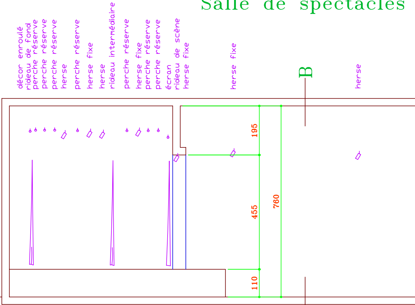
coupe A-A éch. 1/100
