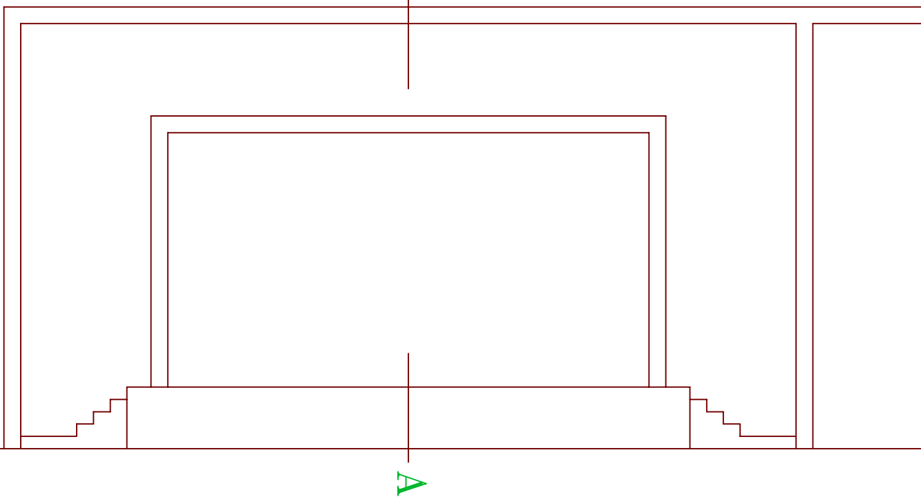
coupe B-B éch. 1/100
