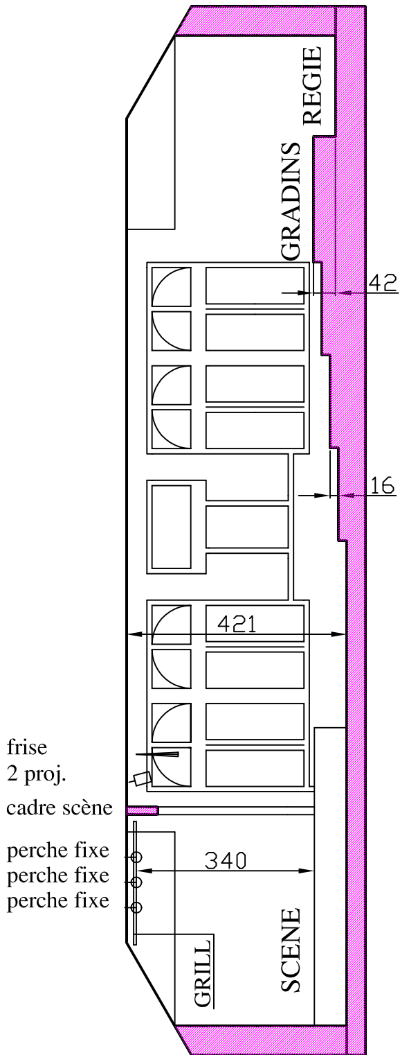
COUPE A - A
