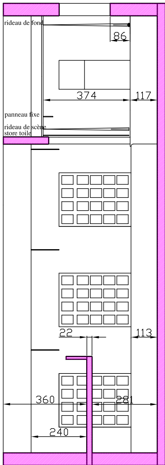
COUPE A - A
