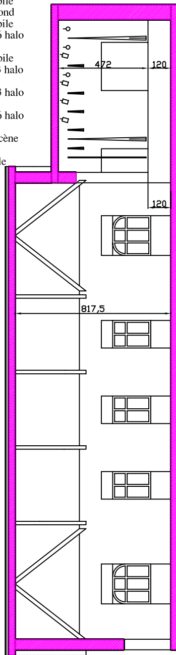
COUPE A - A
