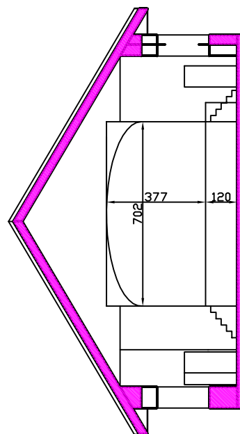
COUPE B - B
