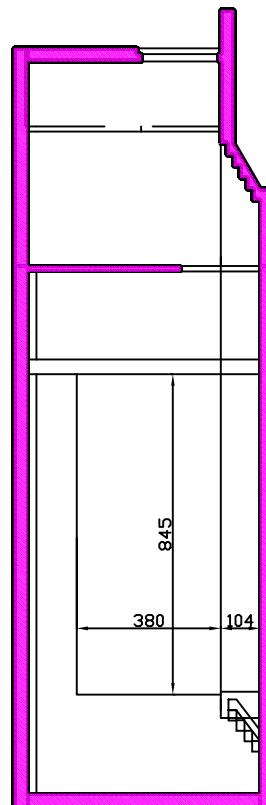
COUPE B - B
