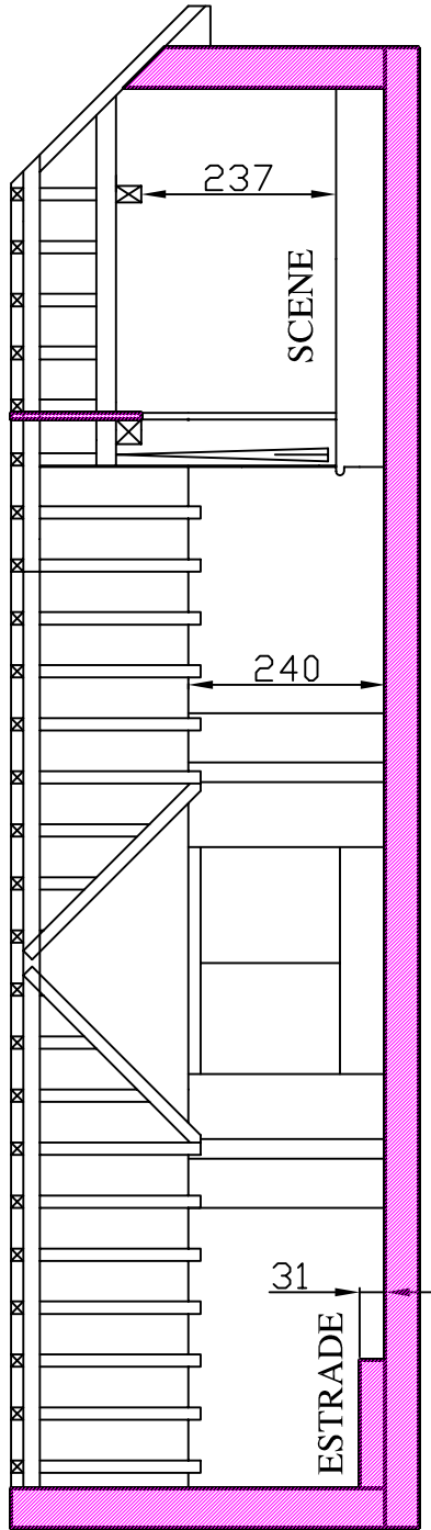
COUPE A - A
