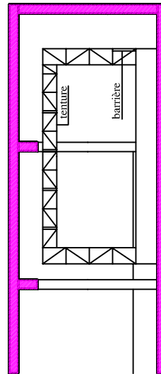
COUPE C - C
