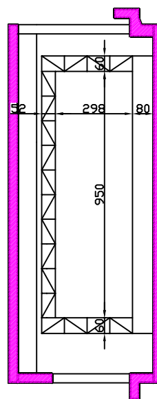
COUPE B - B
