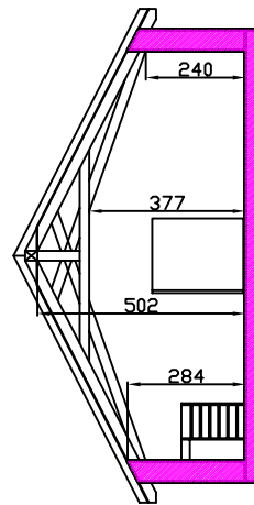
COUPE B - B
