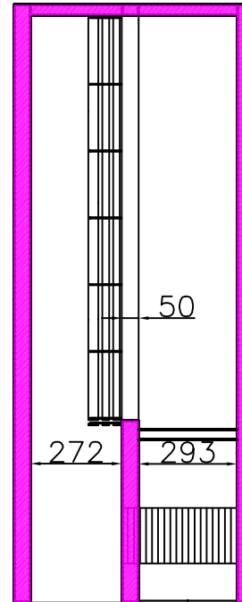
COUPE B - B
