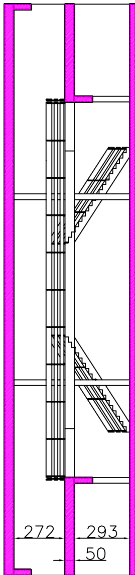
COUPE A - A
