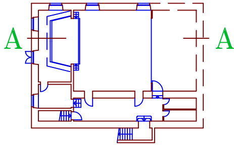
plan éch. 1/500
