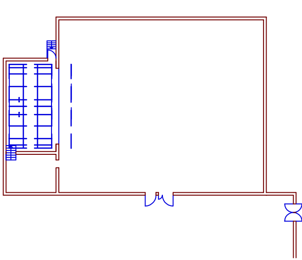
plan éch. 1/500
