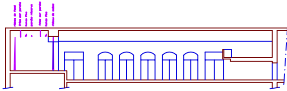
coupe A-A éch. 1/500
