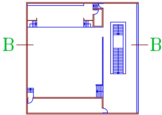
plan éch. 1/500
