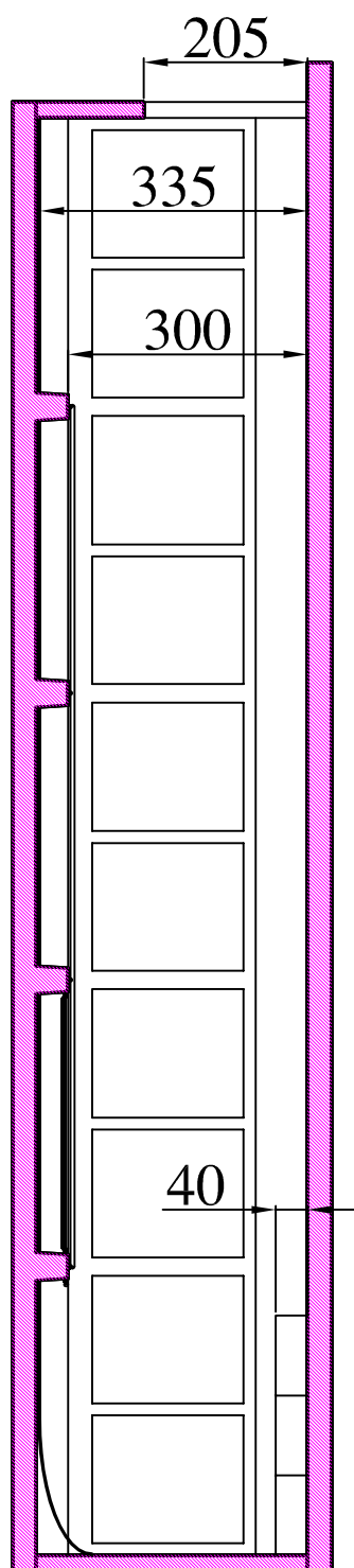
COUPE A - A
